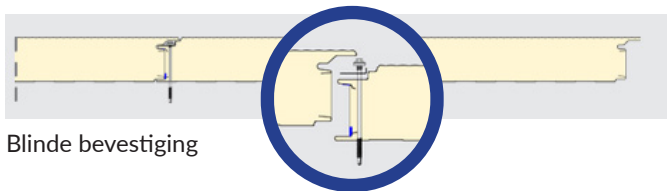
Daktoepassing
